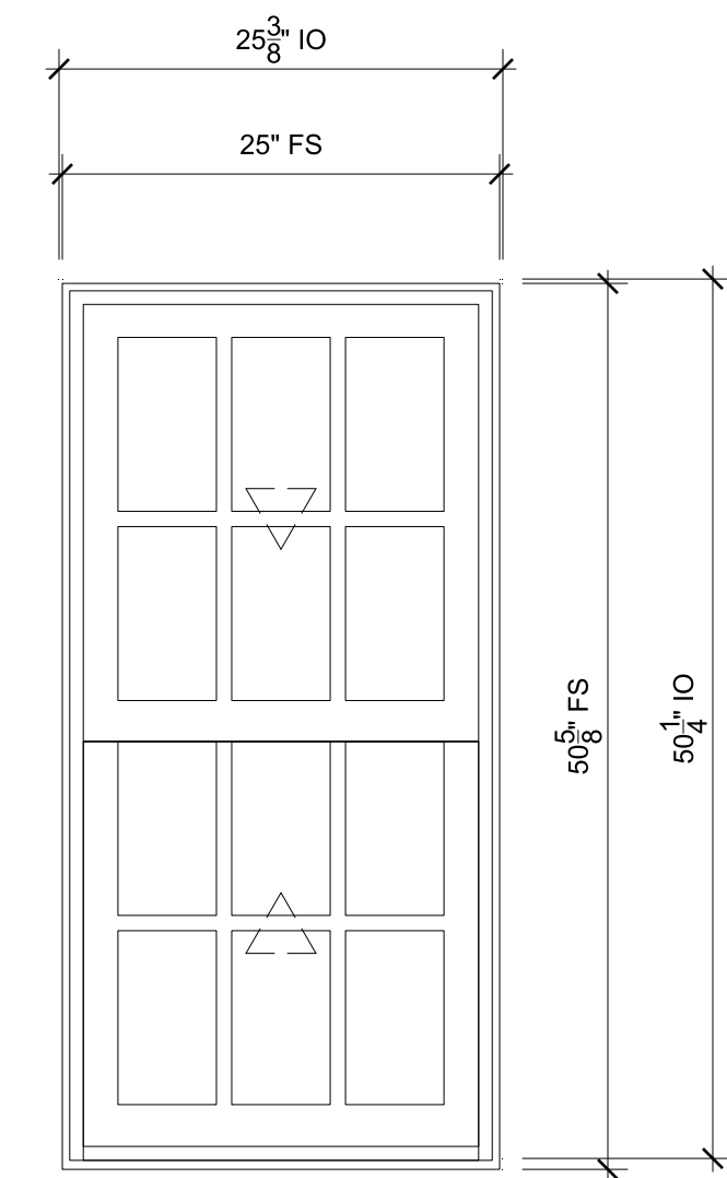
MAIN FLR - SIDE ELE SCALE: 1" = 1'-0"
