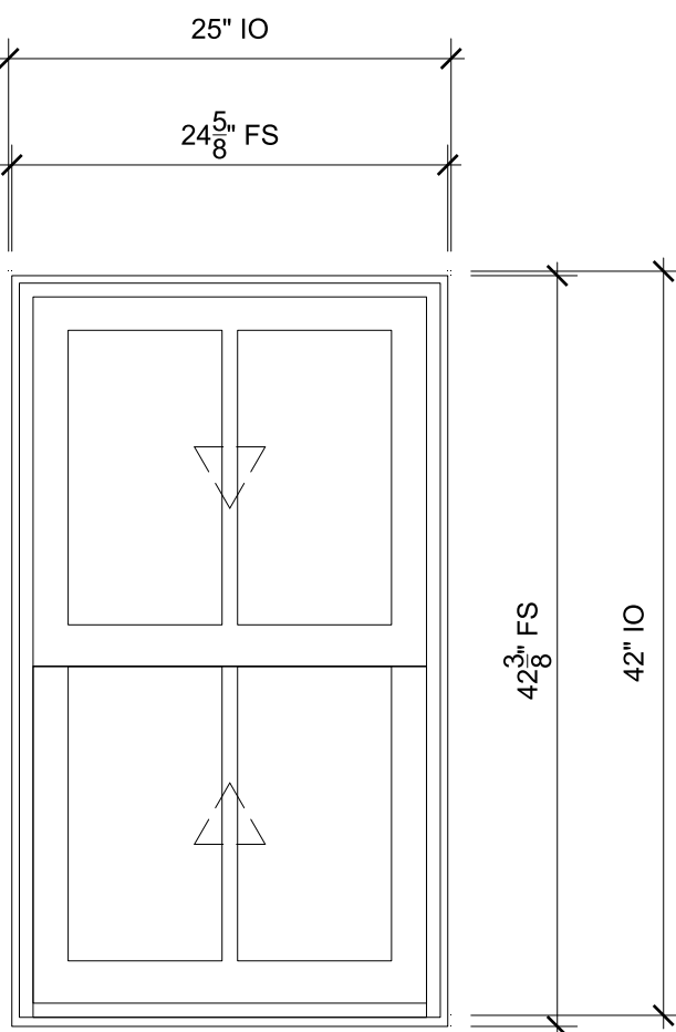
QTY2- SECOND FLR- SIDE ELE SCALE: 1" = 1'-0"
